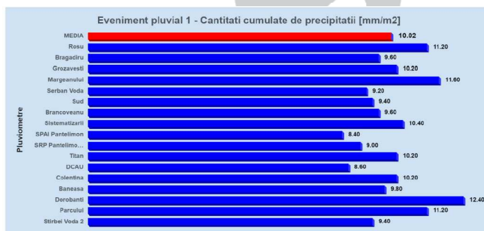
Cantitati de precipitatii totale cumulate in intervalul orar: 14.05.2019 11:30 – 16:30 (5h)
