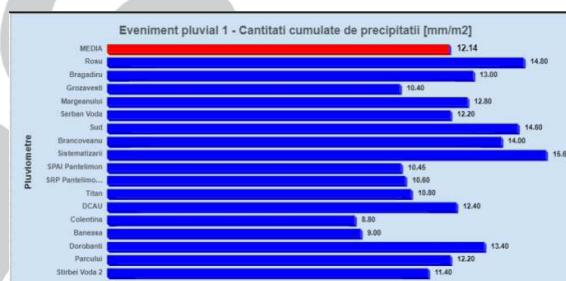
Cantitati cumulate de precipitatii in intervalul orar 06/05/2019 16:20 – 22:30
