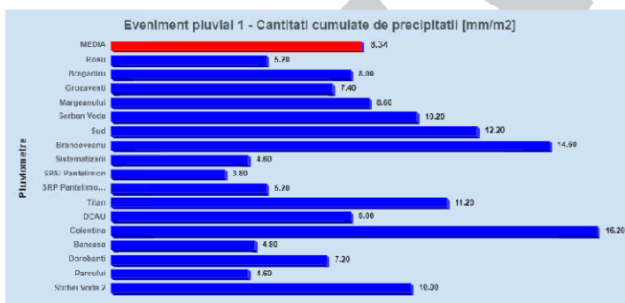
Cantitati de precipitatii total cumulate in intervalul orar: 20.05.2019 18:50 – 21:00
