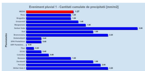
Cantitati cumulate de precipitatii in intervalul orar: 06/05/2019 12:00 – 15:00
